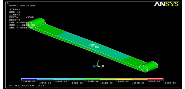
Fig: MASTER LEAF
