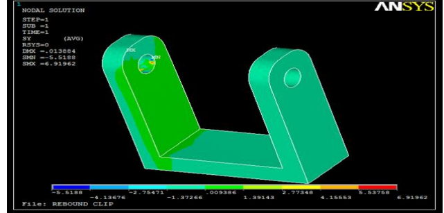
Fig: REBOUND CLIP
